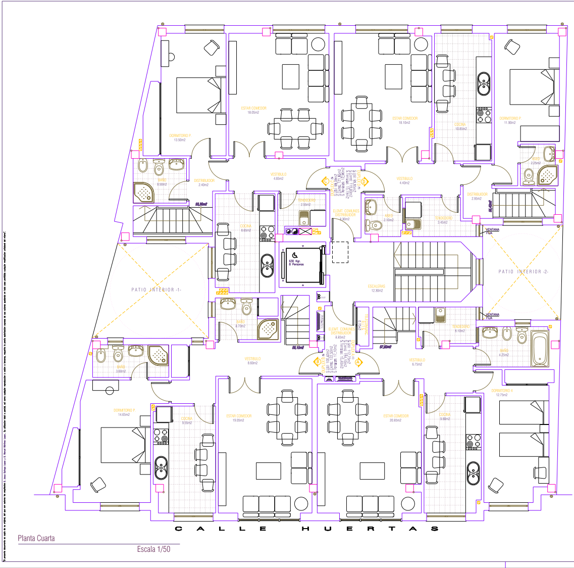
DISTRIBUCION. Planta Cuarta.
