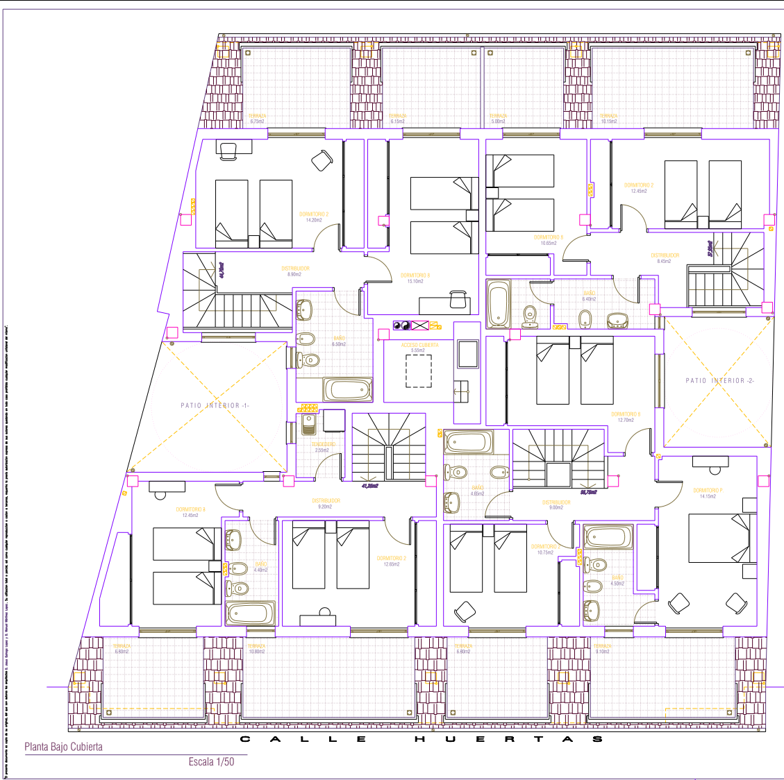
DISTRIBUCION. Planta Bajo Cubierta.
