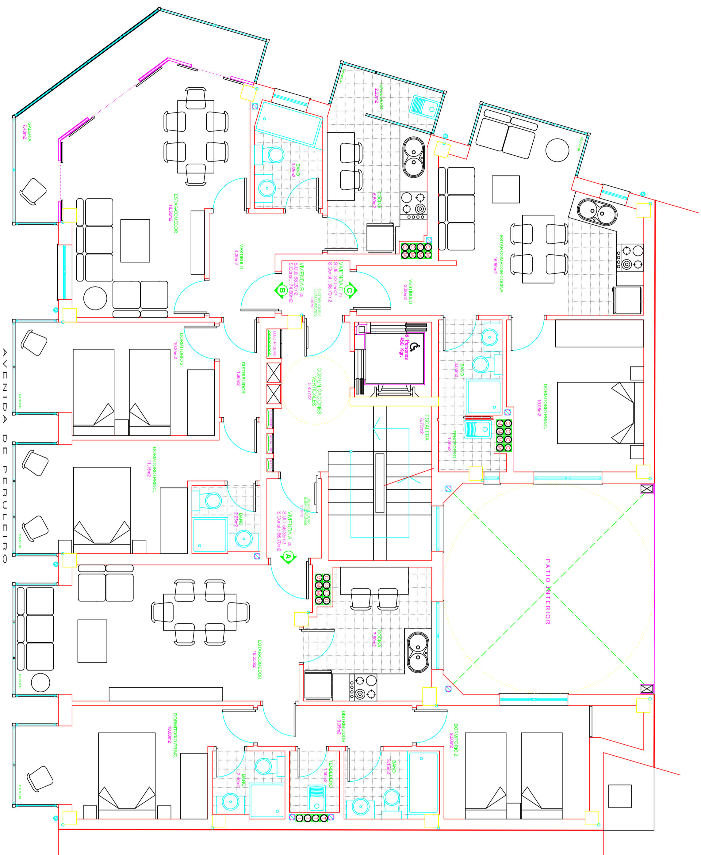
DISTRIBUCION. Plantas Segunda, Tercera, Cuarta y Quinta.
